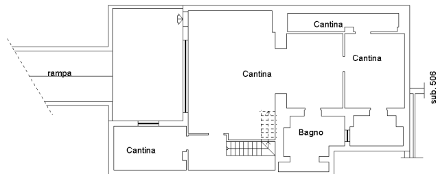
PLANIMETRIA PIANO INTERRATO H. 2,70 M.
