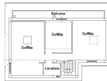
PLANIMETRIA PIANO PRIMO (SOTTOTETTO) H. 2,20 M.
